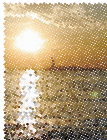
(d) 2557 points
